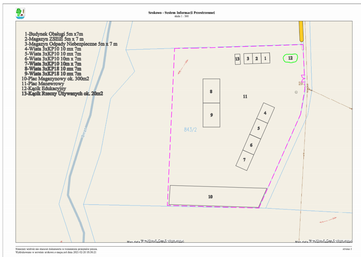
Rysunek 6. Przykładowy układ funkcjonalny punktu
